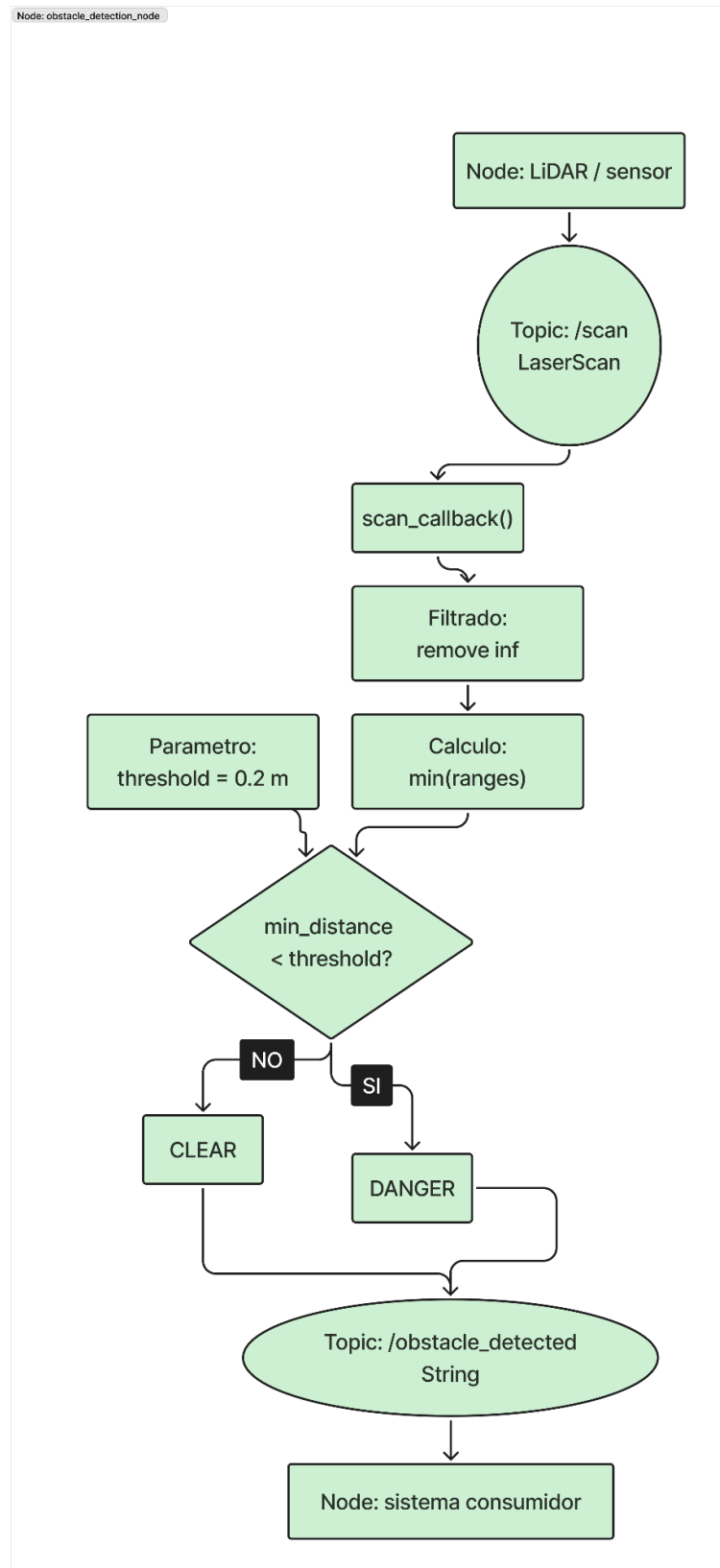
Figura : Diseño de paquete LiDAR
