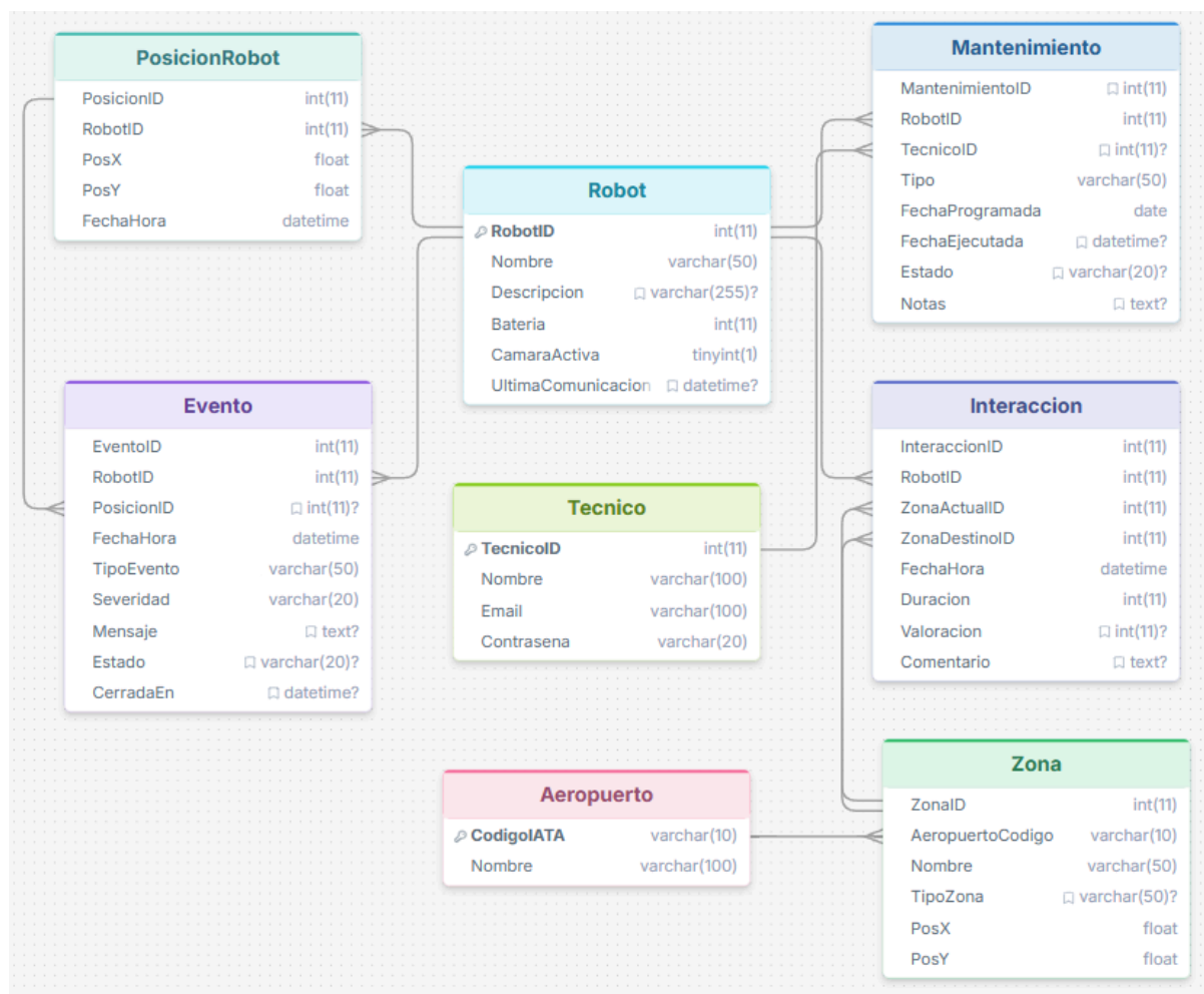
Figura: BBDD
