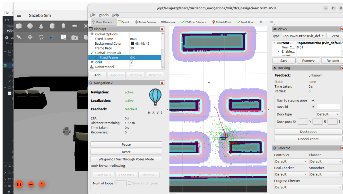
Figuras : Navegación
