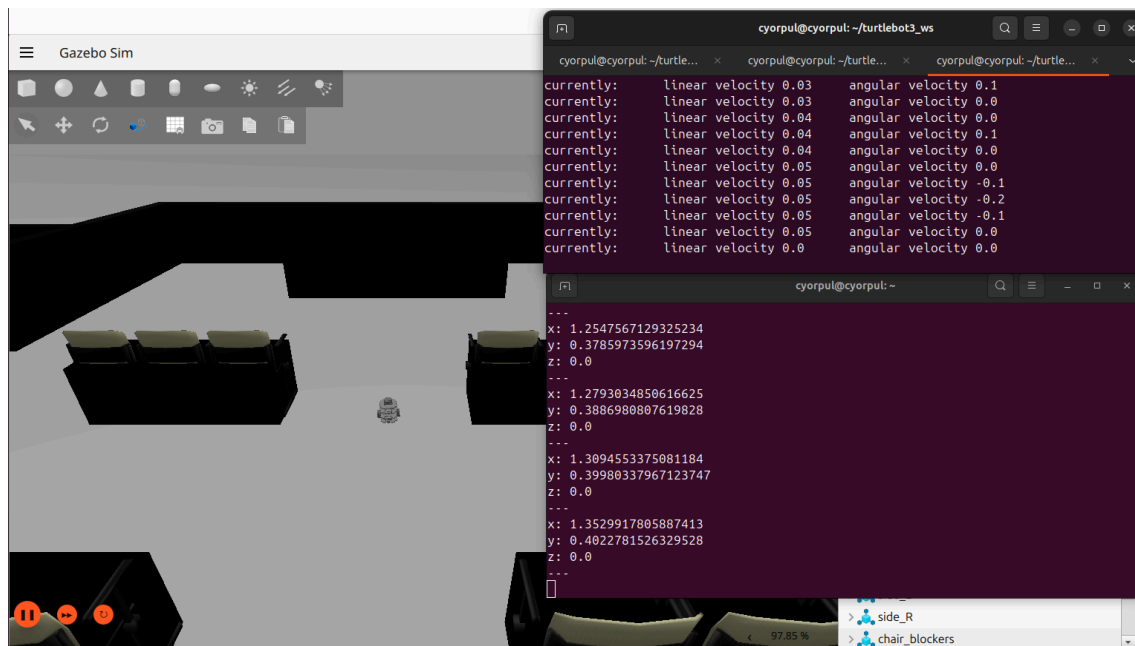
Figuras : Localización
