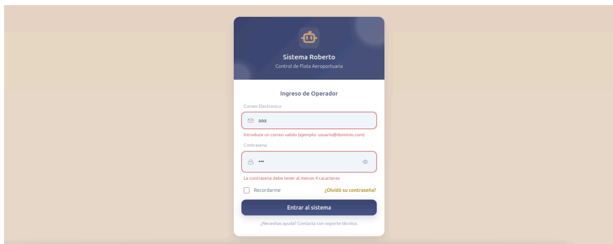
Figura : Login
