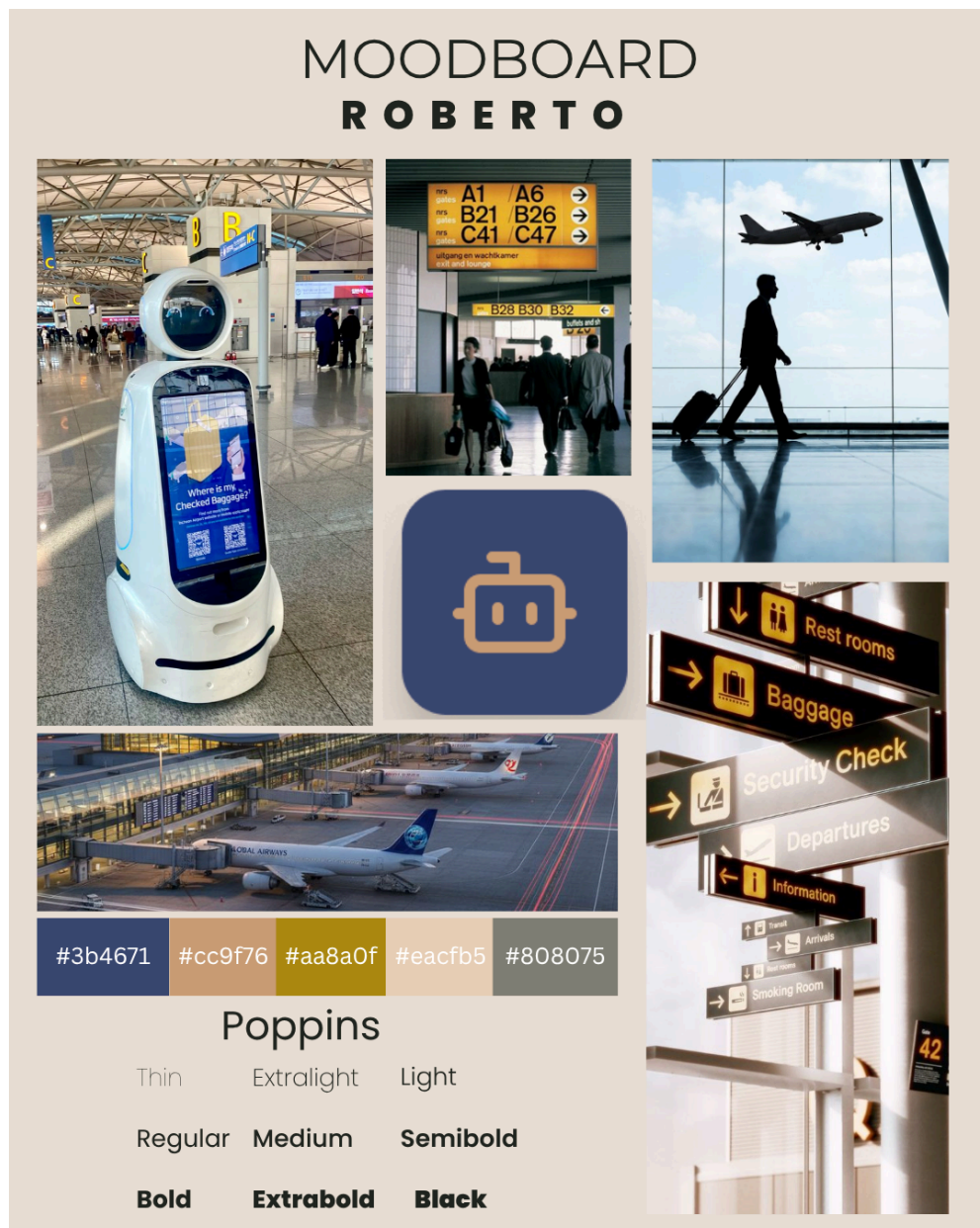
Figura : MoodBoard
